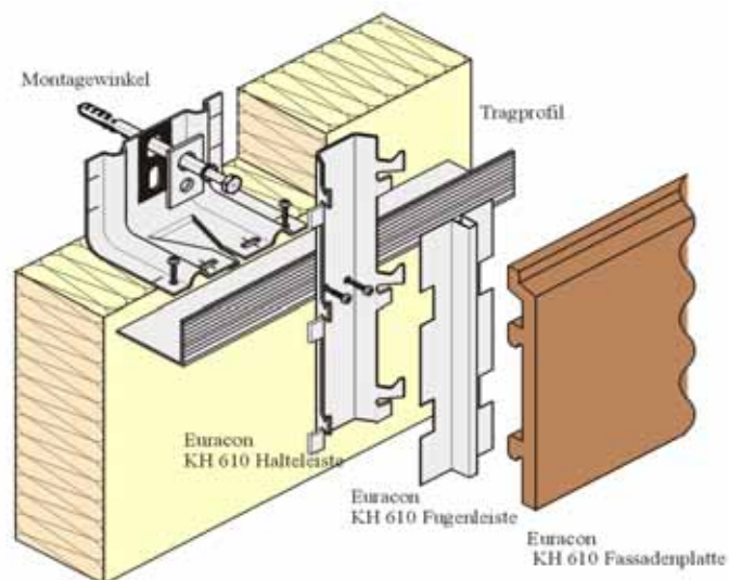
Montageschema: Vorgehängte Keramik-Fassade EURACON KH-610
